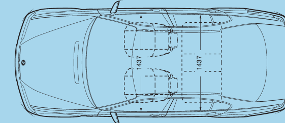
Tutte le misure dei disegni tecnici sono espresse in millimetri. I valori in ( ) si riferiscono alle 316i e 318i; i valori in [ ] alle vetture con trazione integrale. Capacità del bagagliaio 440 litri (misurazione VDA).
