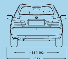
Tutte le misure dei disegni tecnici sono espresse in millimetri. I valori in ( ) si riferiscono alle 316i e 318i; i valori in [ ] alle vetture con trazione integrale. Capacità del bagagliaio 440 litri (misurazione VDA).
